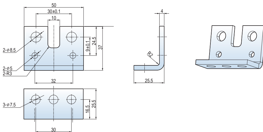
Соединительная шина TD160 4t
